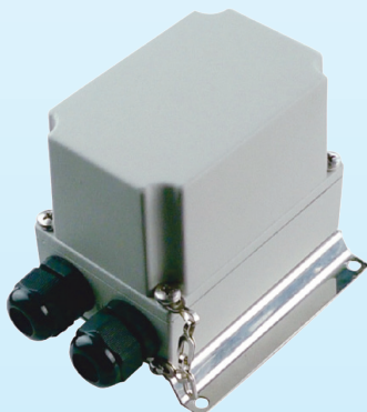
Exemple de montage en commande de deux câbles chauffants d'un modèle Y1B2P, combiné avec un boîtier Y29
